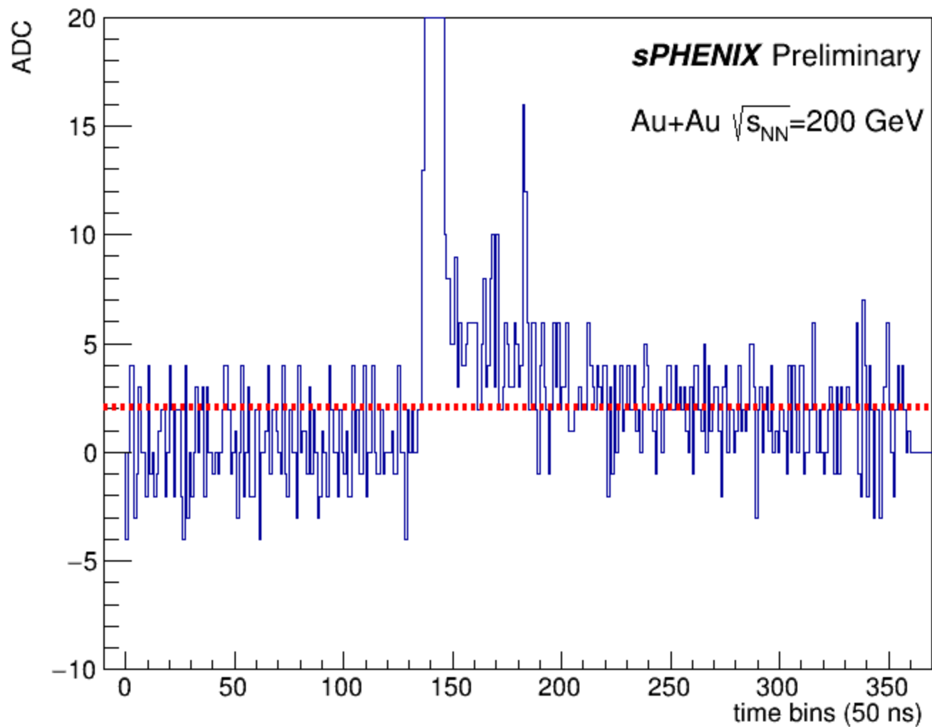
ADC vs time R2 sec08 fee12 Chan74 event0 (400<ADC<600)
