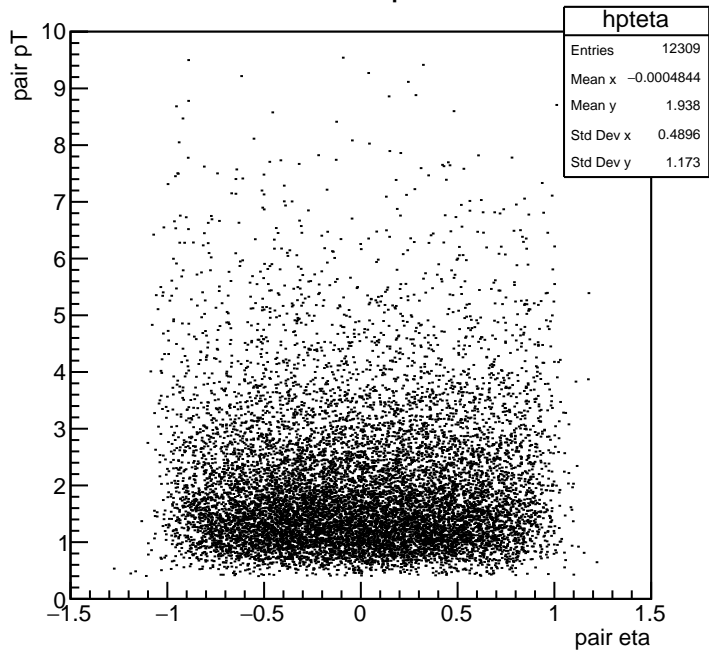
eta vs pT
