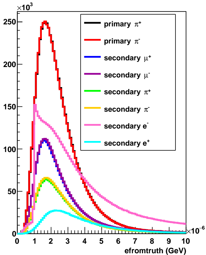
cluster e
