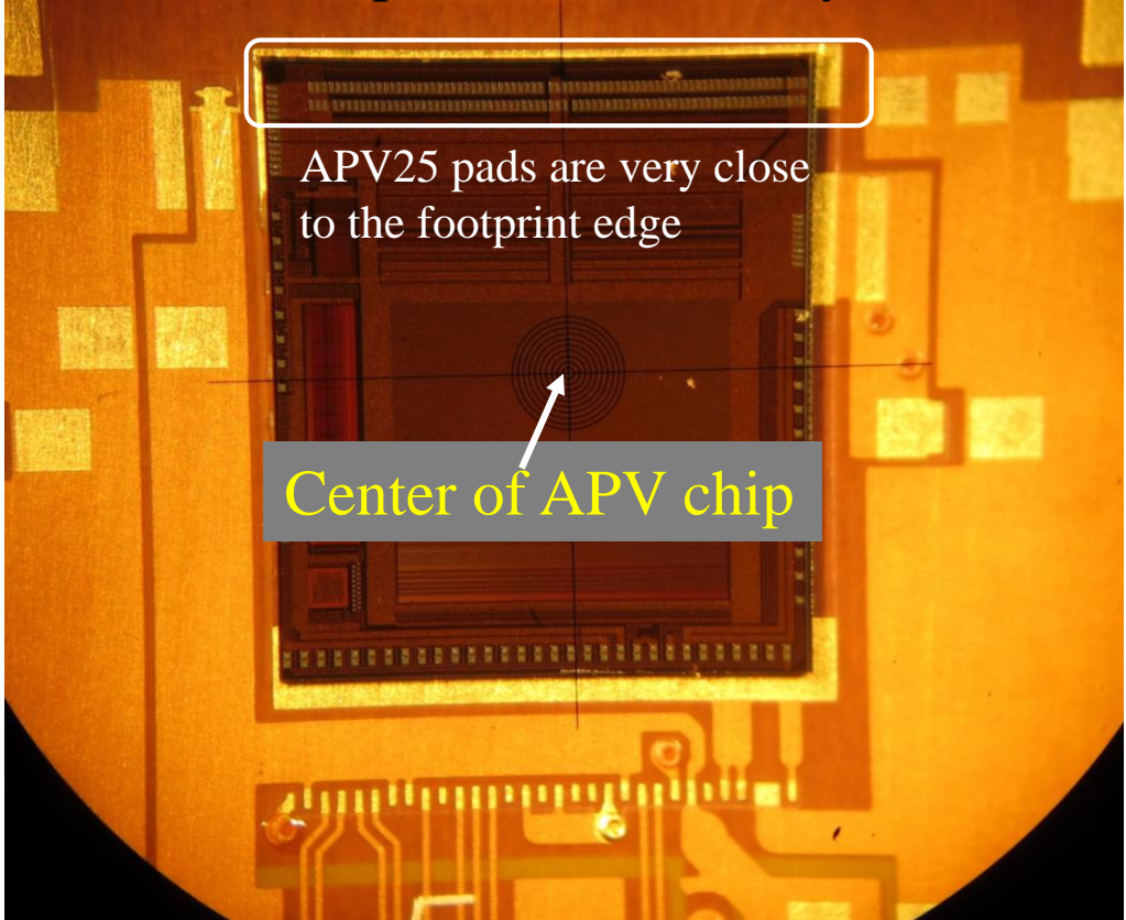
An APV25 chip assembled on hybrid in IST
