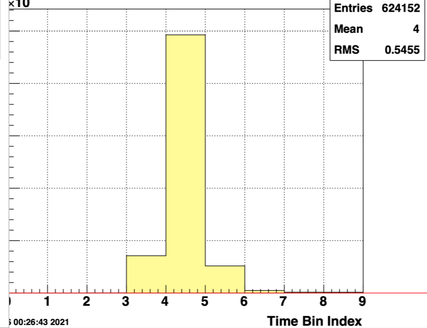
FST - Max ADC Time Bin (ZS)
