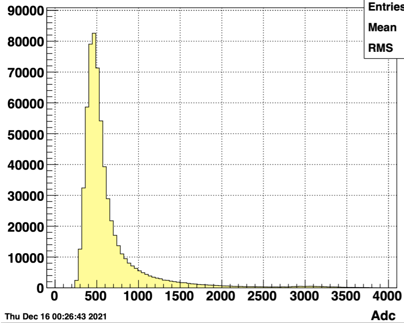
FST - Max ADC (ZS)
