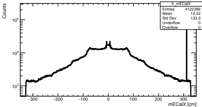
ECaIX (Global)
