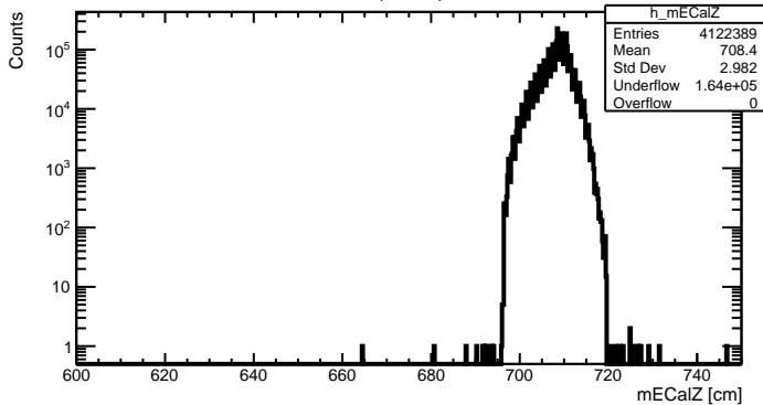
ECalZ (Global)
