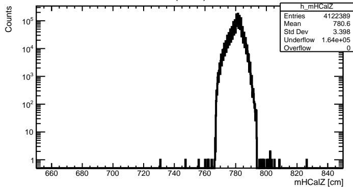
HCalZ (Global)
