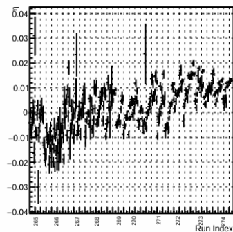
Dev track eta
