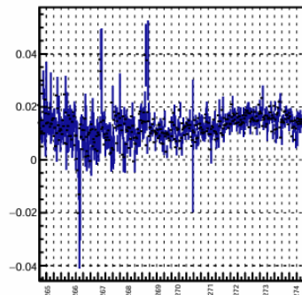
Average full jet eta
