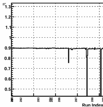
Dev track eta
