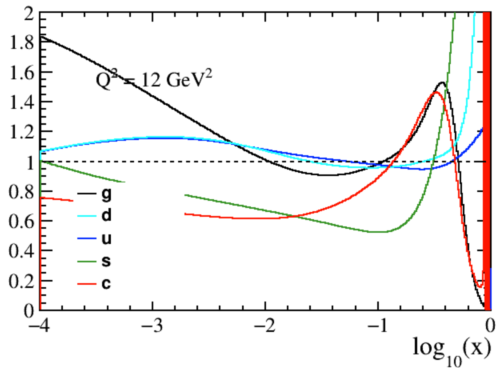
NP2DF2.3 L0 QCD+QED/CTEQ6L
