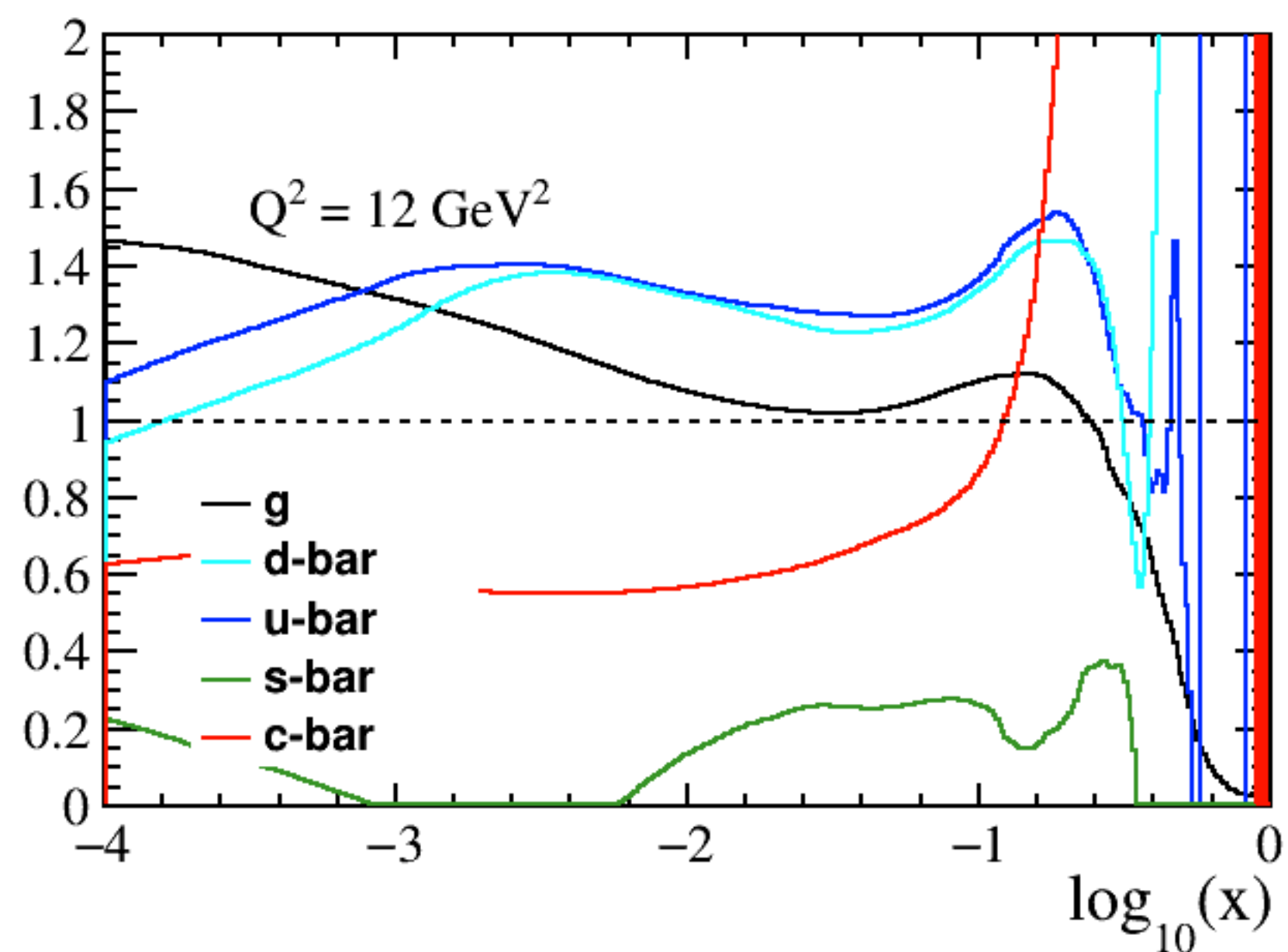
NNPDF3.1 L0 QCD/CTEQ6L
